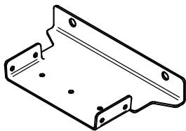
SUPPORT LATÉRAL INFÉRIEUR (G) BOTTOM SIDE BRACKET 2X PL77328
