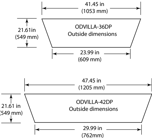
Drain Pan ODVILLA-36DP ODVILLA-42DP
