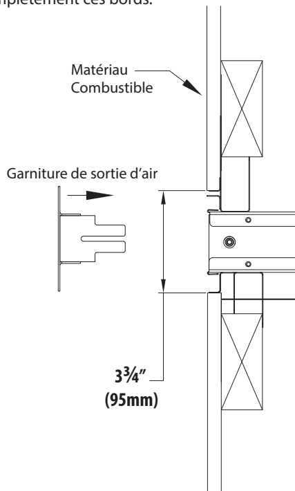
Figure 3.5, Revêtement en matériau combustible
