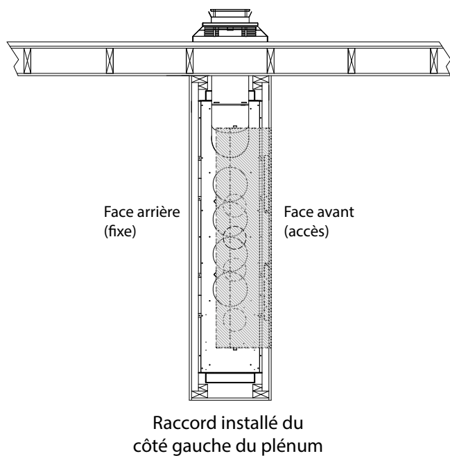
#KZK-054 sortie murale à l'avant
