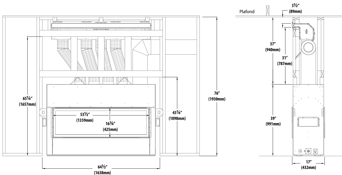
Figure 2.9, Dégagements et dimensions minimum d'encadrement de plénum pour le foyer CLW-ST
