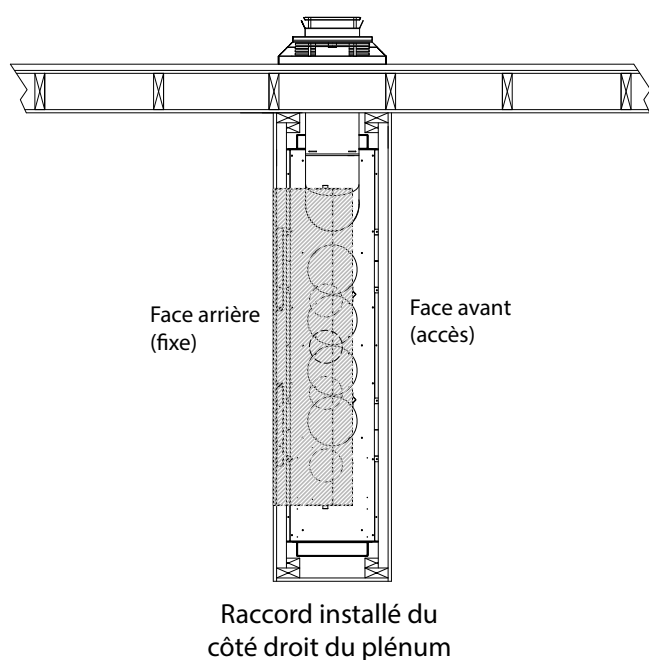
#KZK-054 sortie murale à l'arrière
