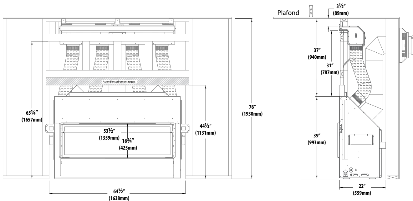
Figure 2.8, Dégagements et dimensions minimum d'encadrement de plénum pour le foyer CLW-50
