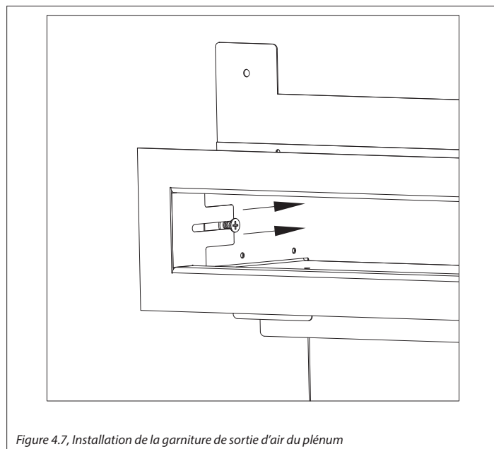
Figure 4.7, Installation de la garniture de sortie d'air du plénum
