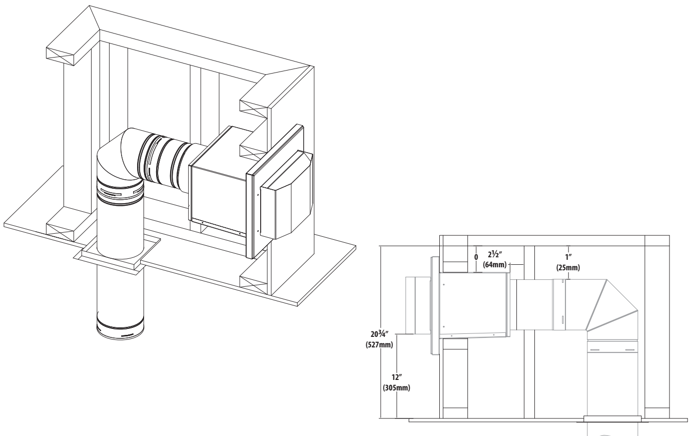
Figure 3.4, Dégagements minimums pour une terminaison au toit
