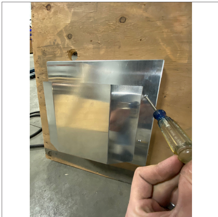
Figure 5.1, Retrait du couvercle avant
