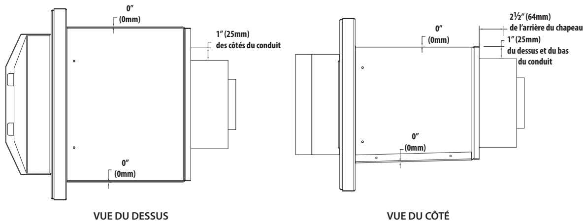
Figure 3.3, Dégagements minimums aux matériaux combustibles
