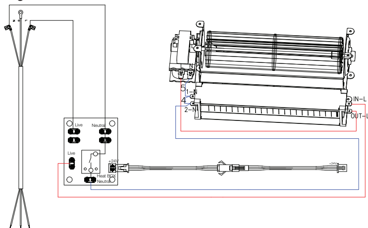
Diagrama del Cableado
