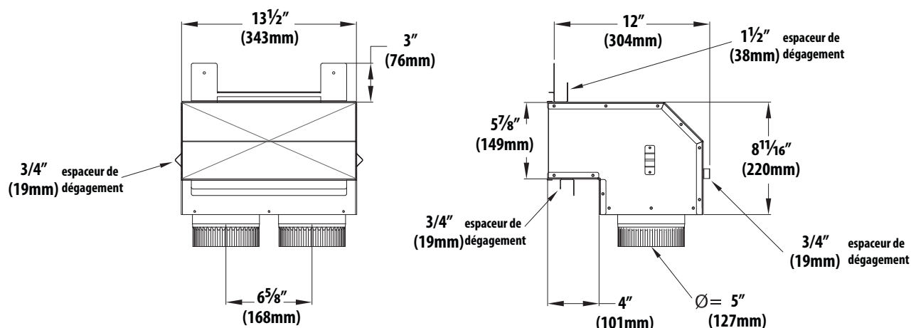
Figure 1.4, Dimensions du KZK-158A
