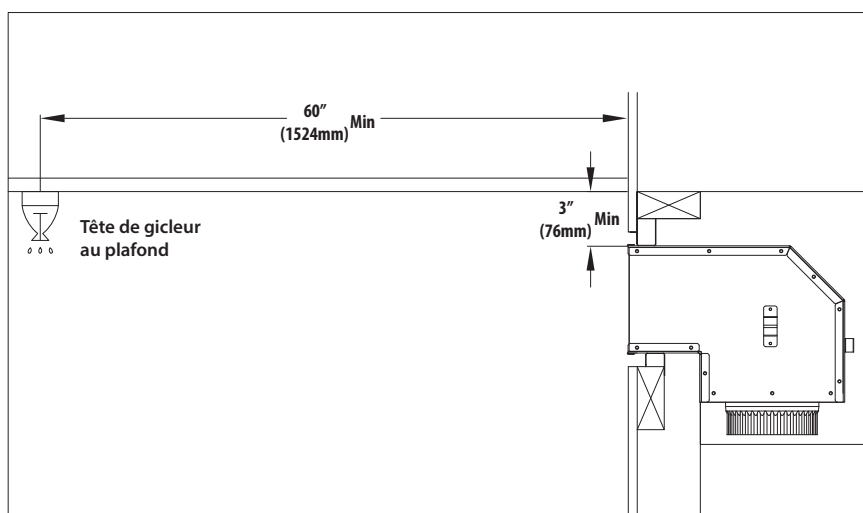
Figure 2.1, Dégagement au gicleur du kit KZK
