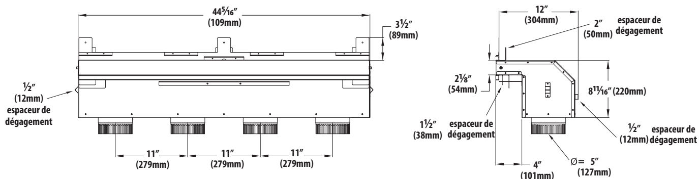
Figure 1.4, Dimensions du KZK-044
