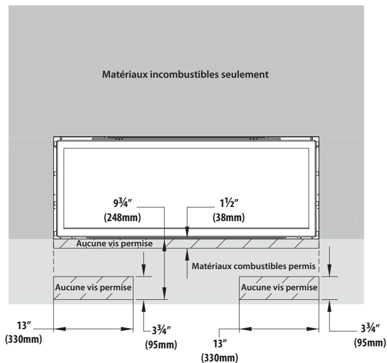
Figure 3.2, Emplacements de vis permis (pour matériaux incombustibles de finition de dimensions minimales)
