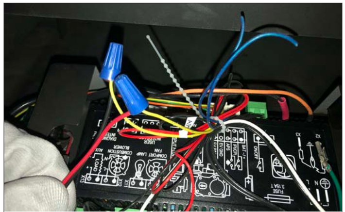
Figure 4.7, Serre-fils installés aux fils identifiés «APS»
