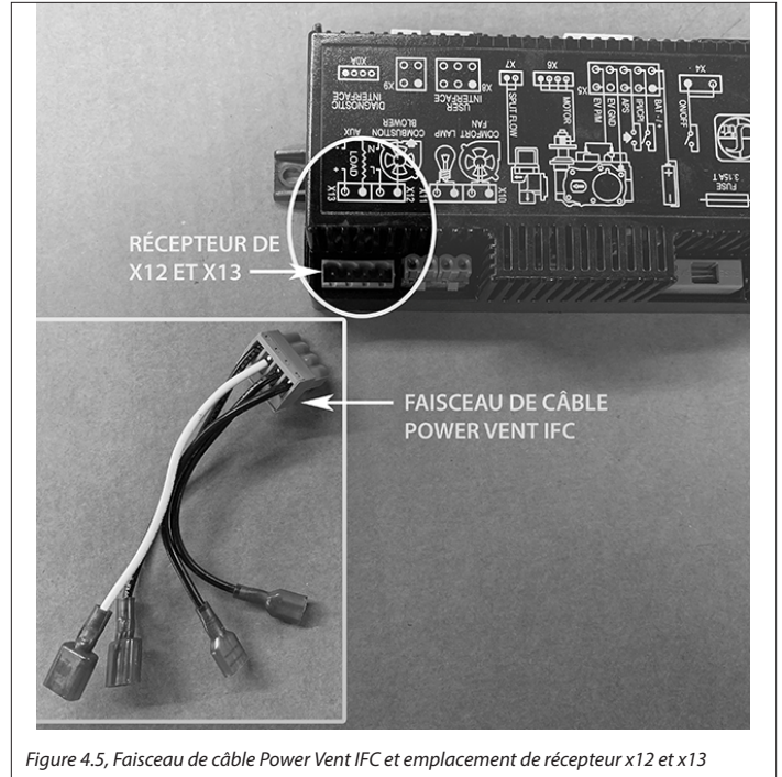
Figure 4.5, Faisceau de câble Power Vent IFC et emplacement de récepteur x12 et x13
