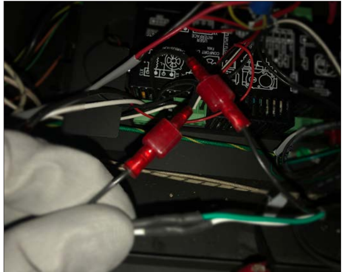
Figure 4.6, Connexion des fils noirs à branchement rapide
