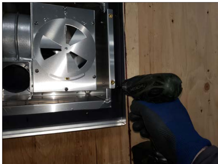
Figure 3.20, Le chapeau est fixé dans le mur
